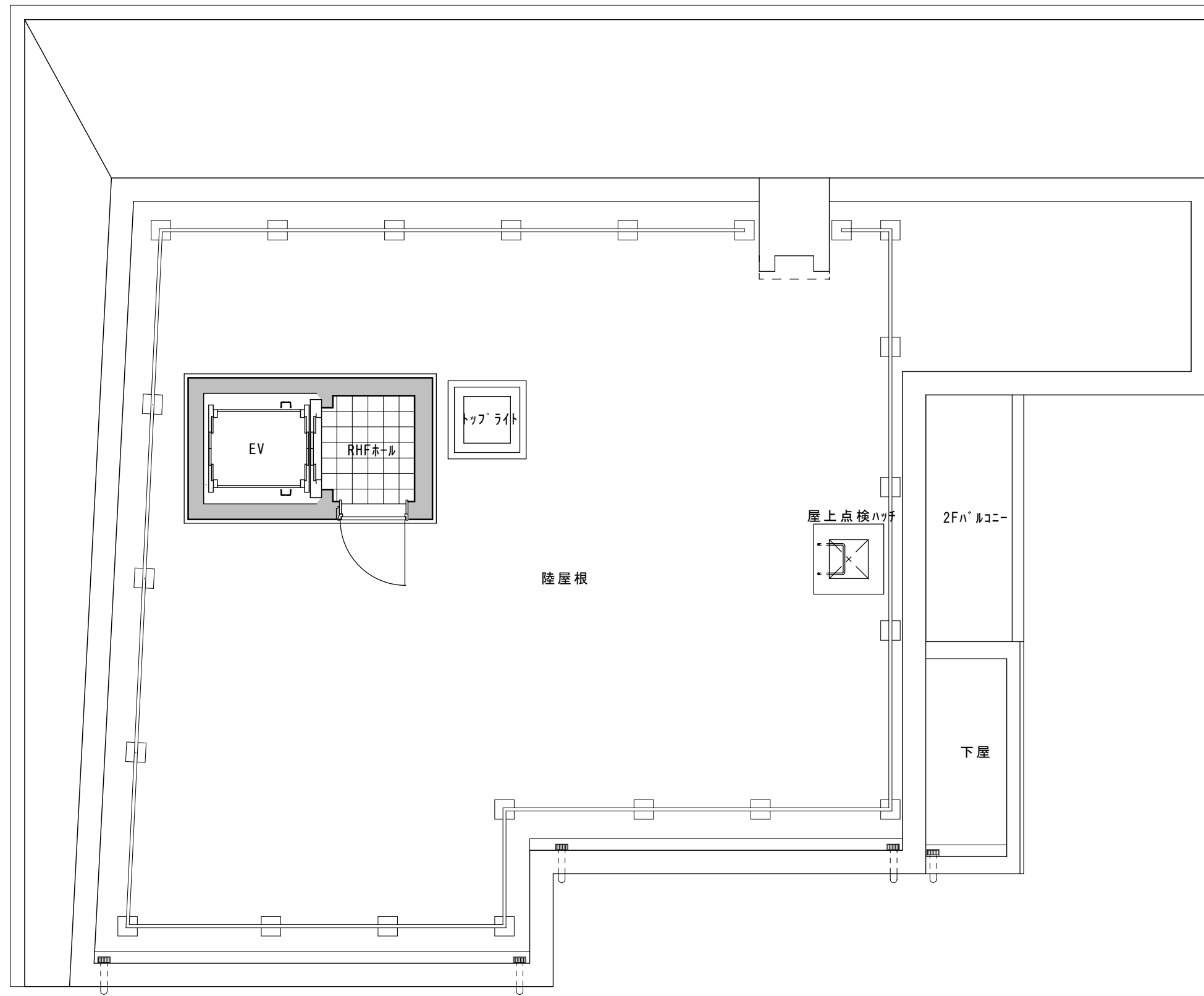
PH階平面図
