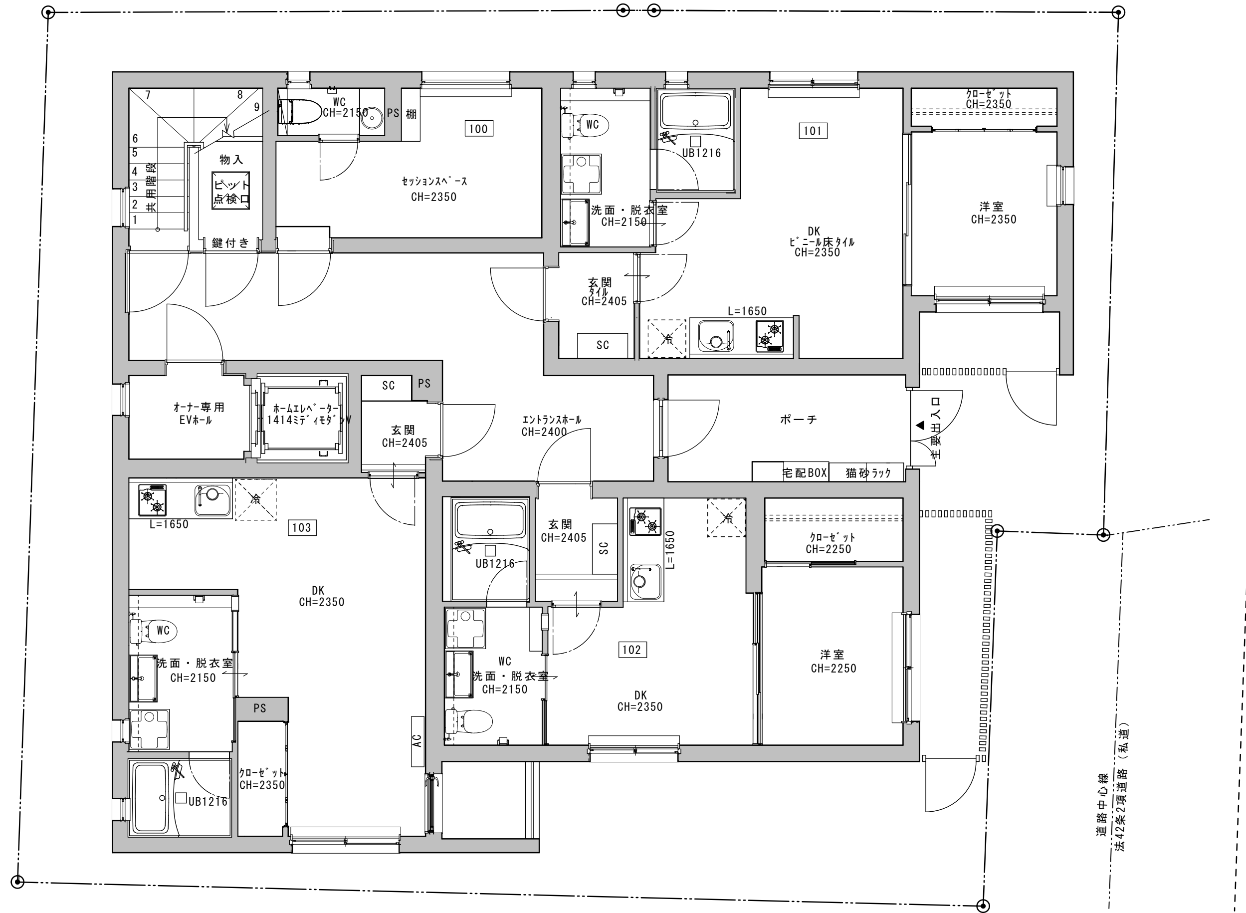
1階平面図
