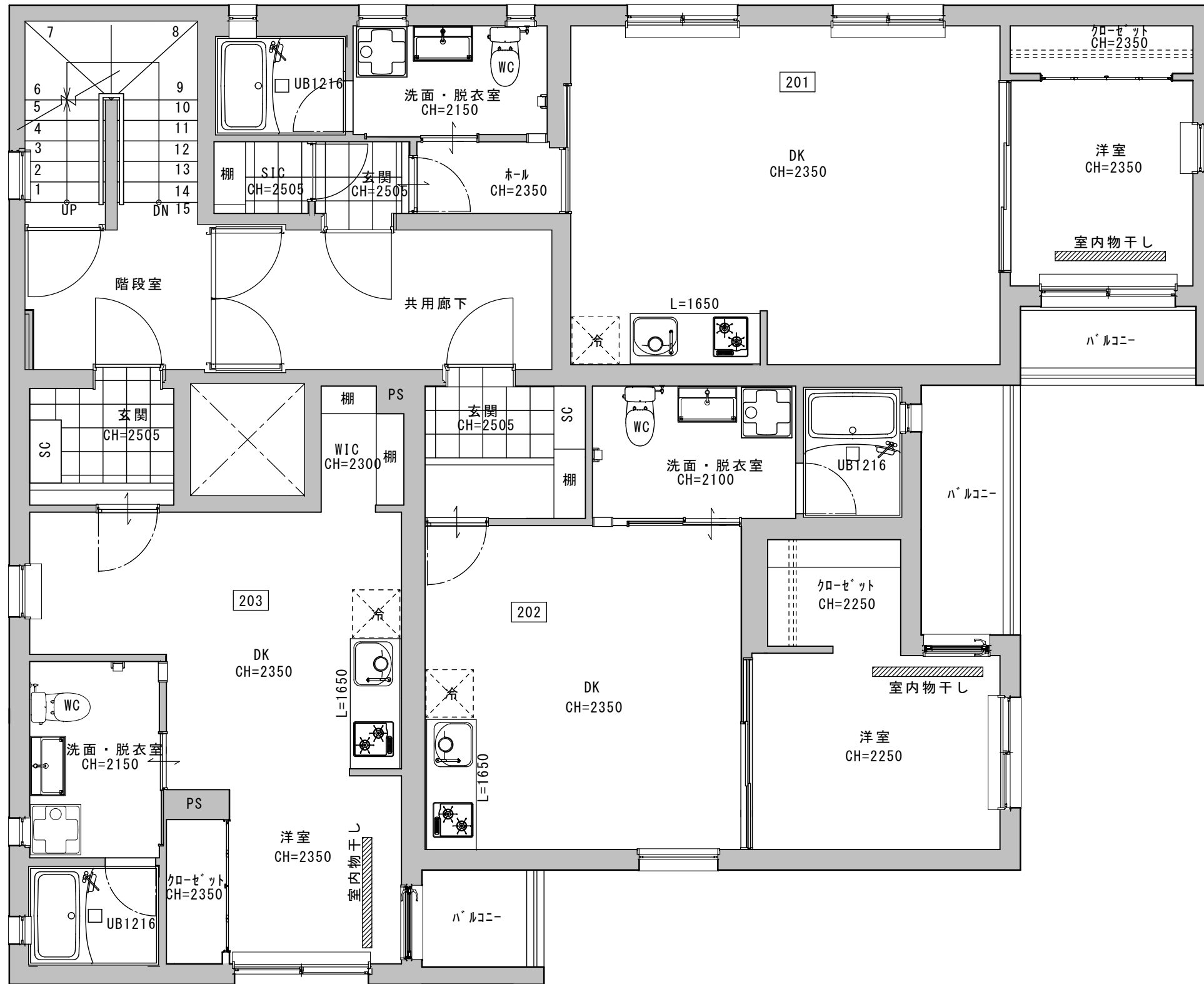
2階平面図
